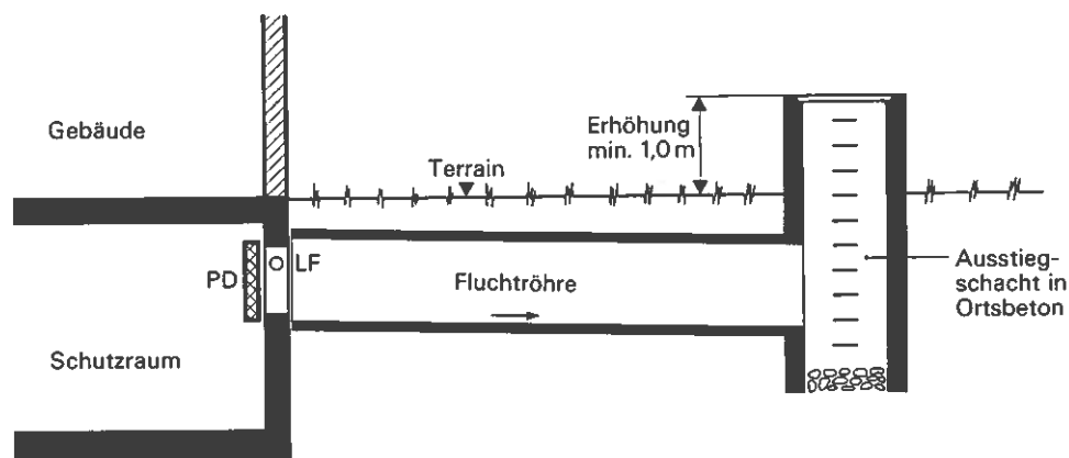
Figur 2.3-1 Fluchtröhre mit erhöhtem Ausstiegschacht
