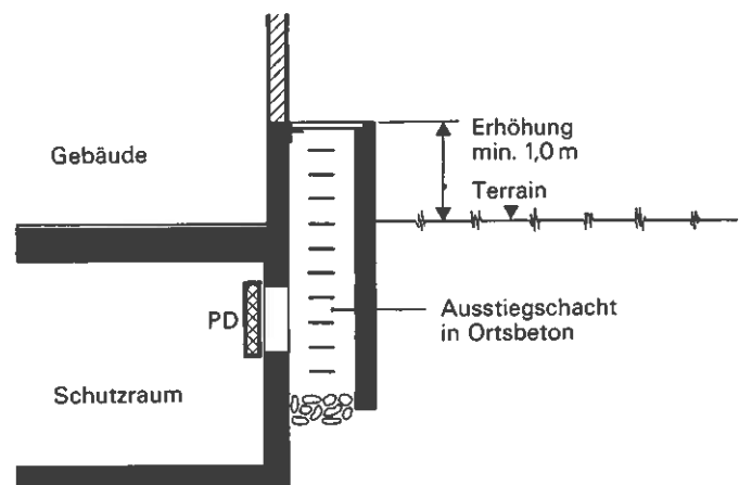
Figur 2.3-2 Notausstieg mit erhöhtem Ausstiegschacht
