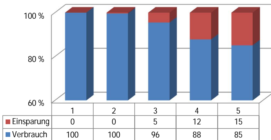
Grafik: Einsparung Strom im AMFZ dank Betriebsoptimierung
