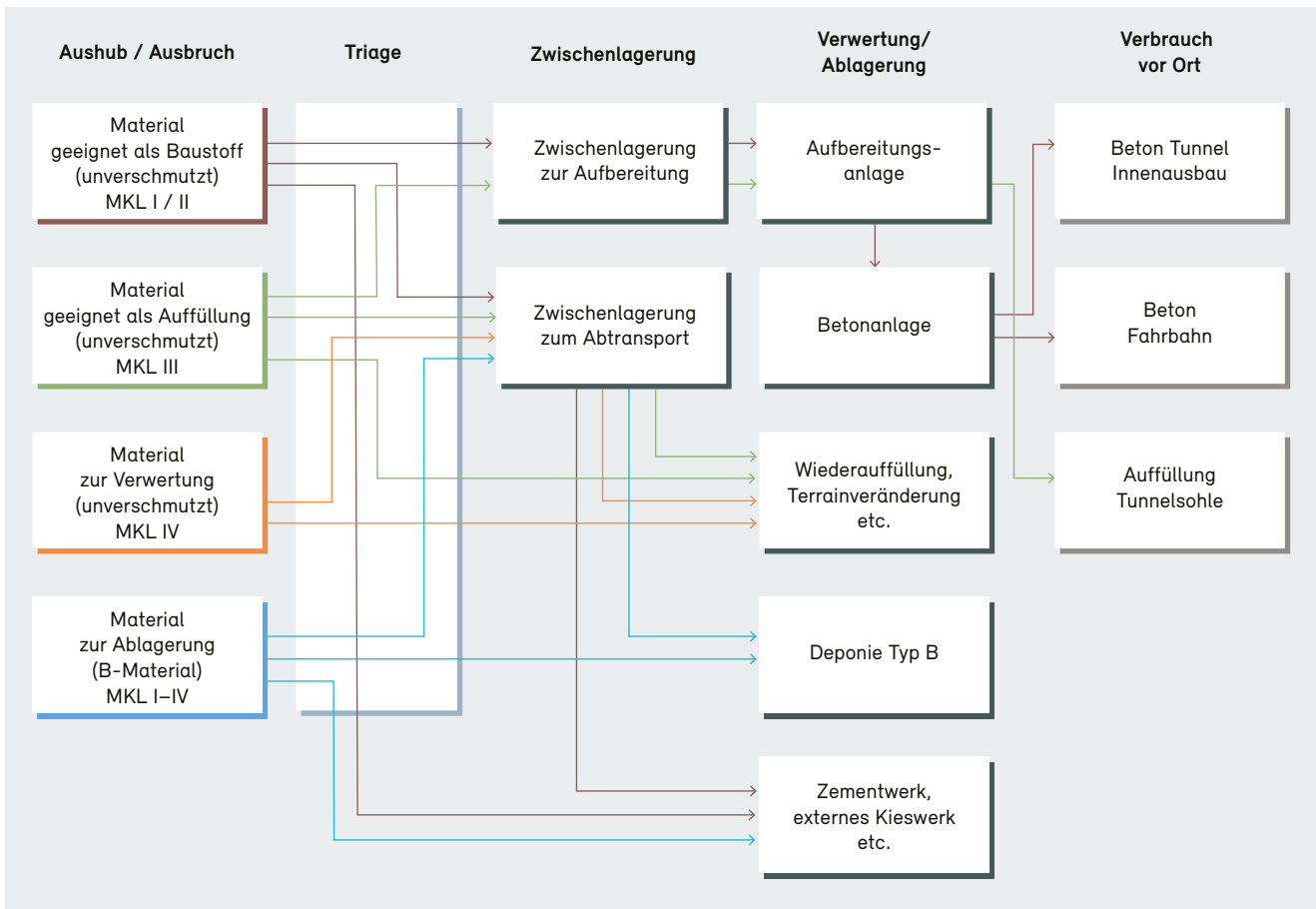
Abbildung A3-5 Beispiel eines Massenflussdiagramms
